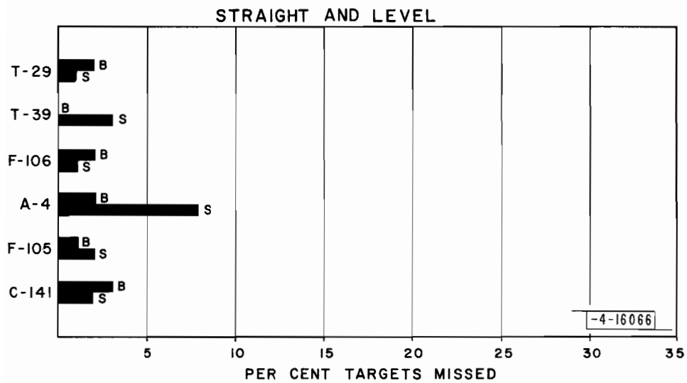
Fig. 17(a). En route miss rates.
