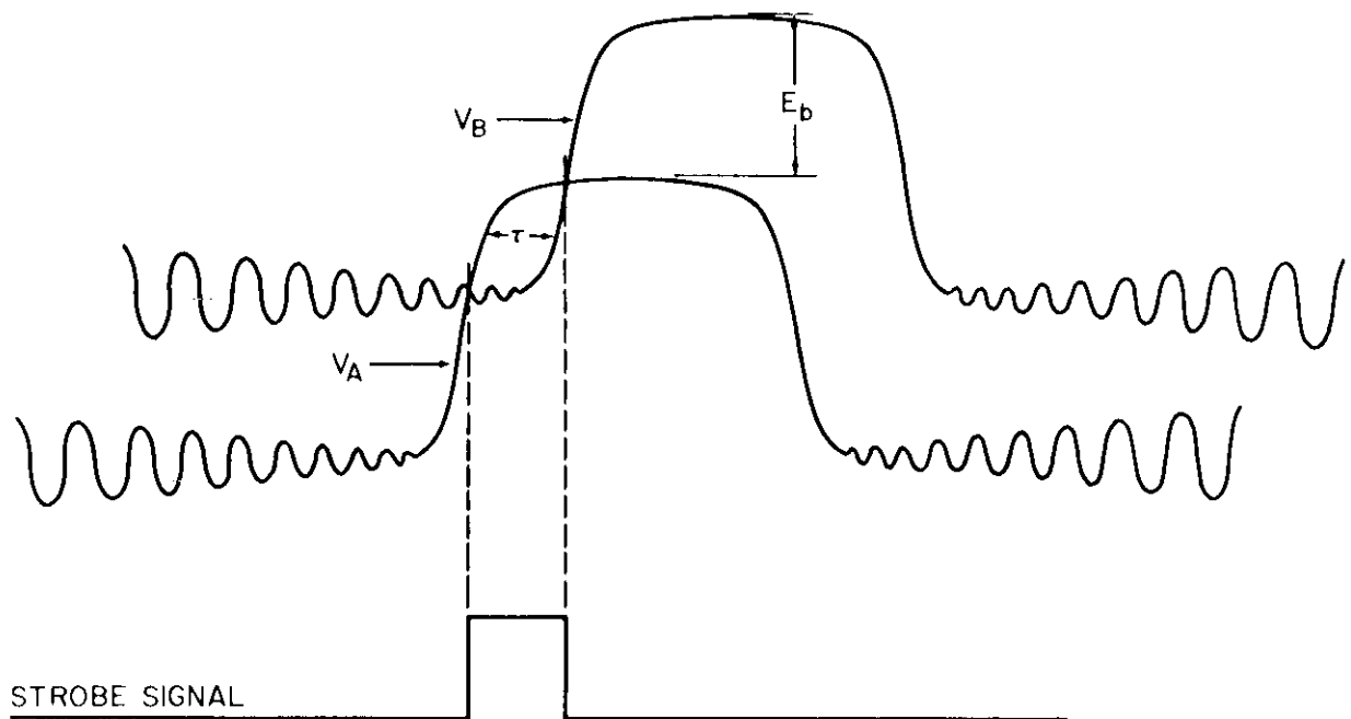
Fig. 29. Log video strobe generator.
